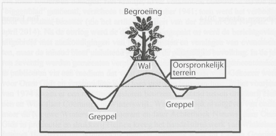
Dwarsdoorsnede van een landweer.
